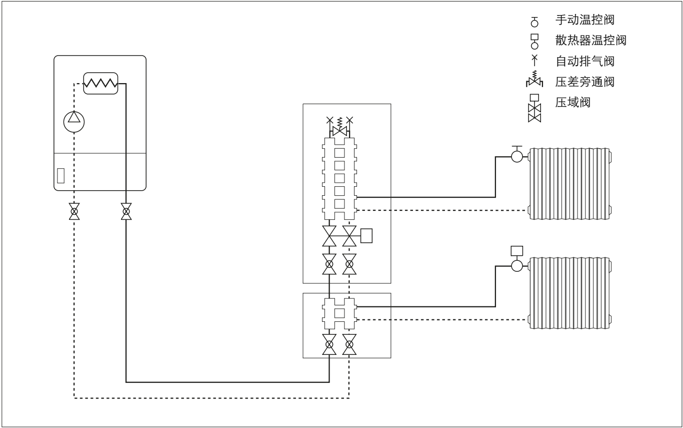
362073+362036分水箱在系统上的运用图示
