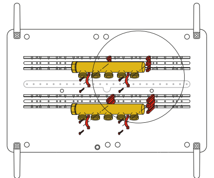
360001型支架安装图示
