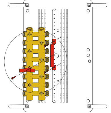
362001型支架安装图示
