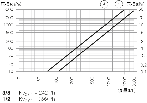
角型手动温控阀，340,411和415型
