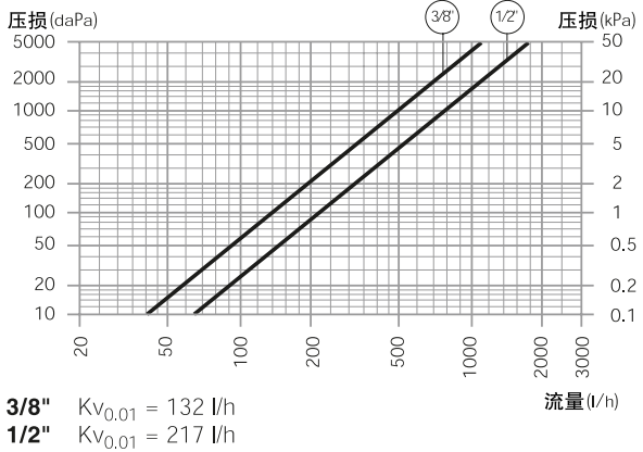
直型手动温控阀，341,412和416型
