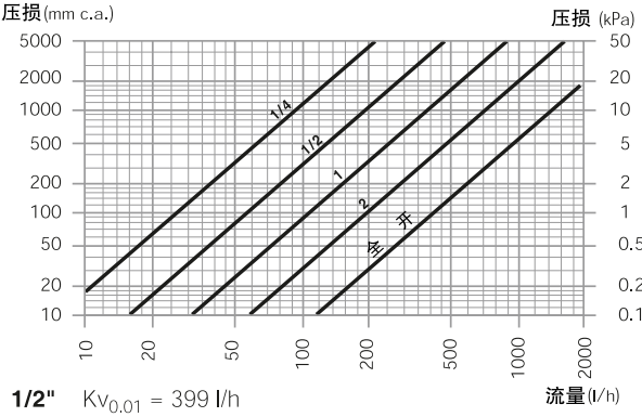
角型回水阀1/2", 342, 431和435型
