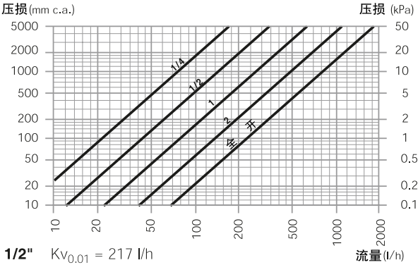
直型回水阀1/2", 343, 432和436型
