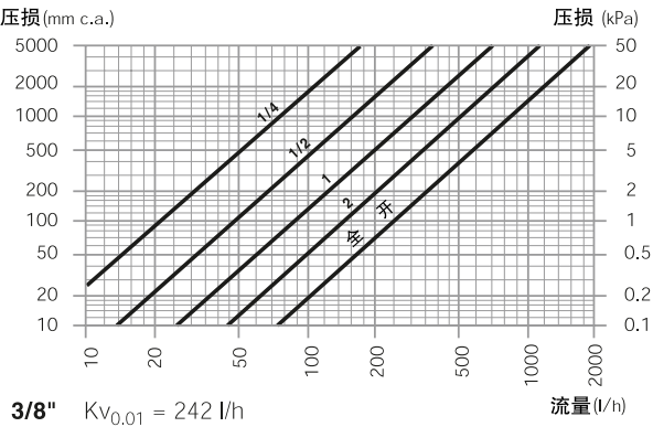
角型回水阀3/8", 342,431和435型
