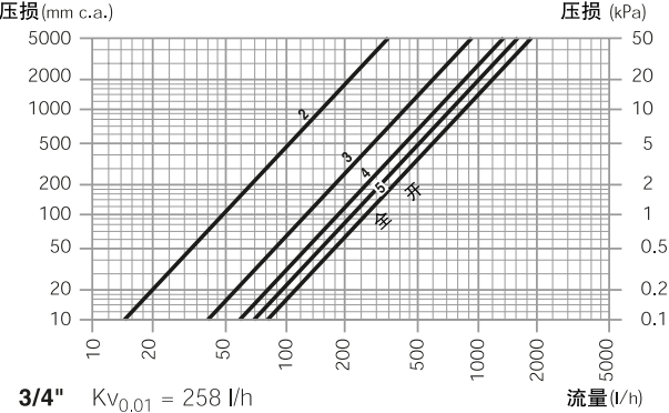
直型回水阀3/4", 432型
