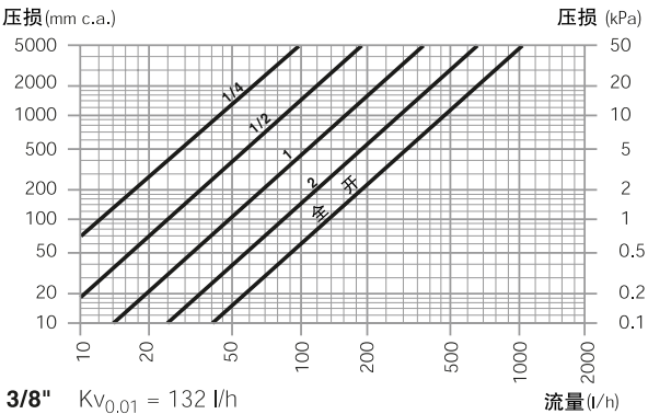
直型回水阀3/8", 343, 432和436型
