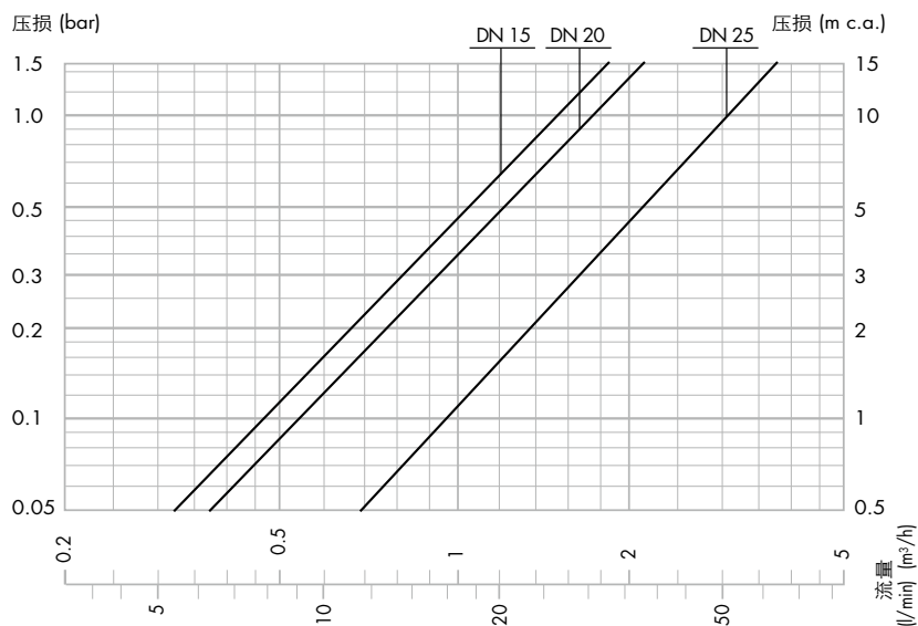
为保证 ±2°C 精确度的建议流量
