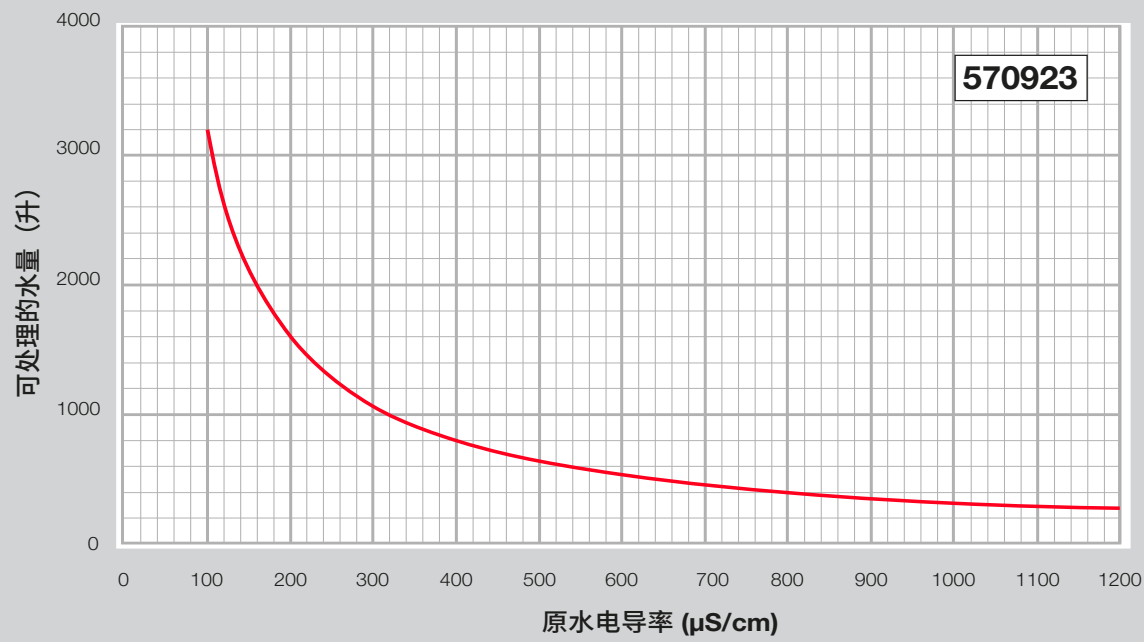
充载式滤芯选型图表
