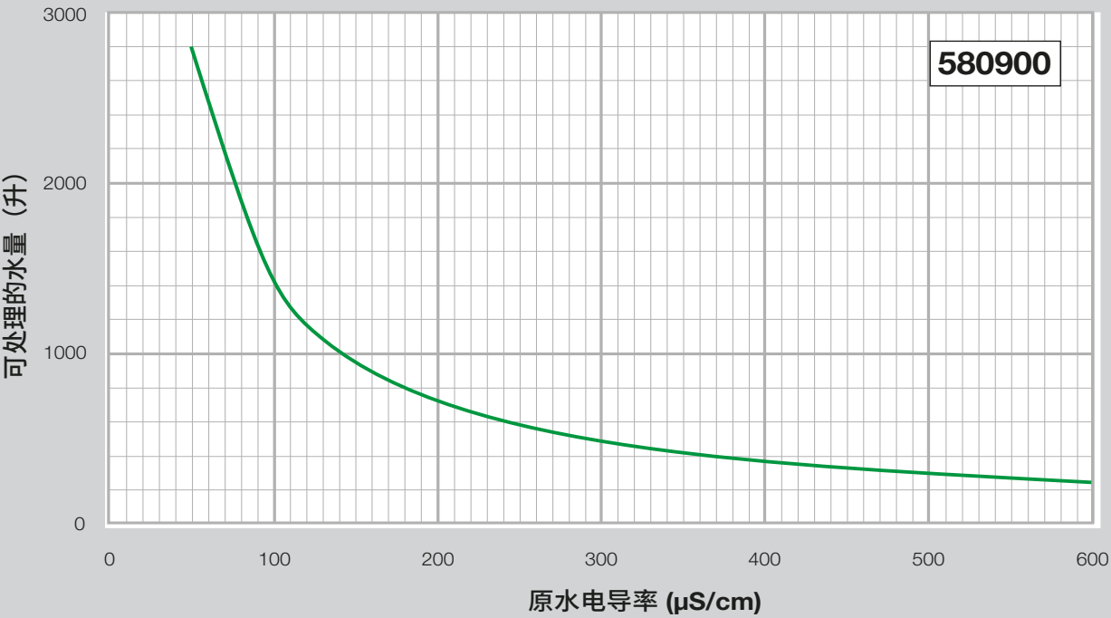
一次性滤芯选型图表
