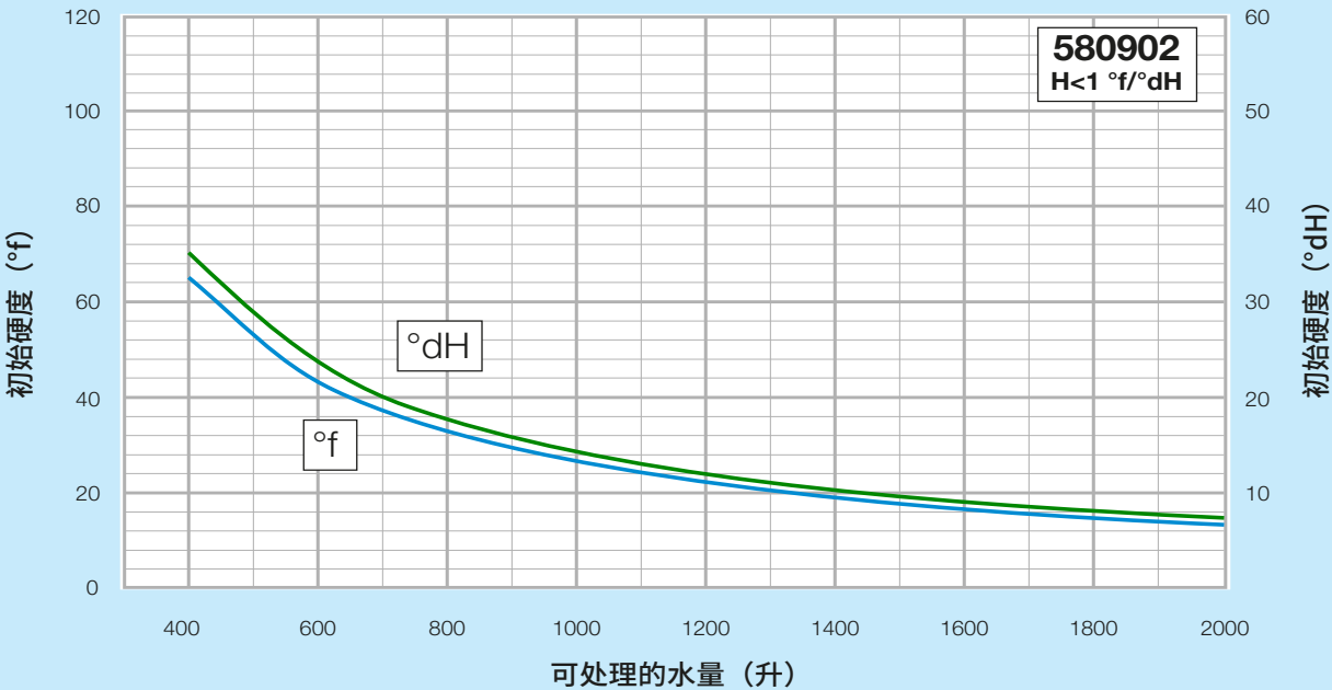
一次性滤芯选型图表
