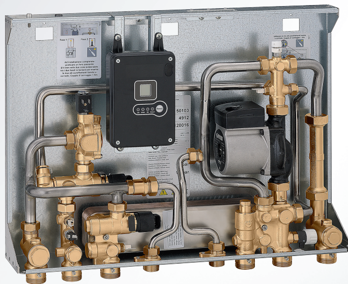
嵌墙式-SATK 50
